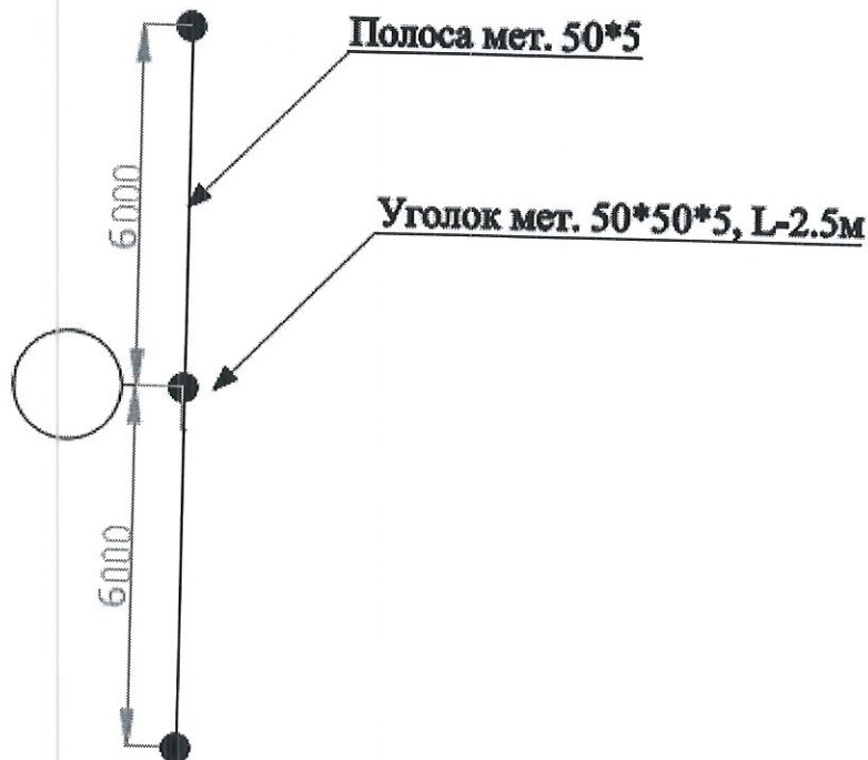
Схема заземляющего устройства
